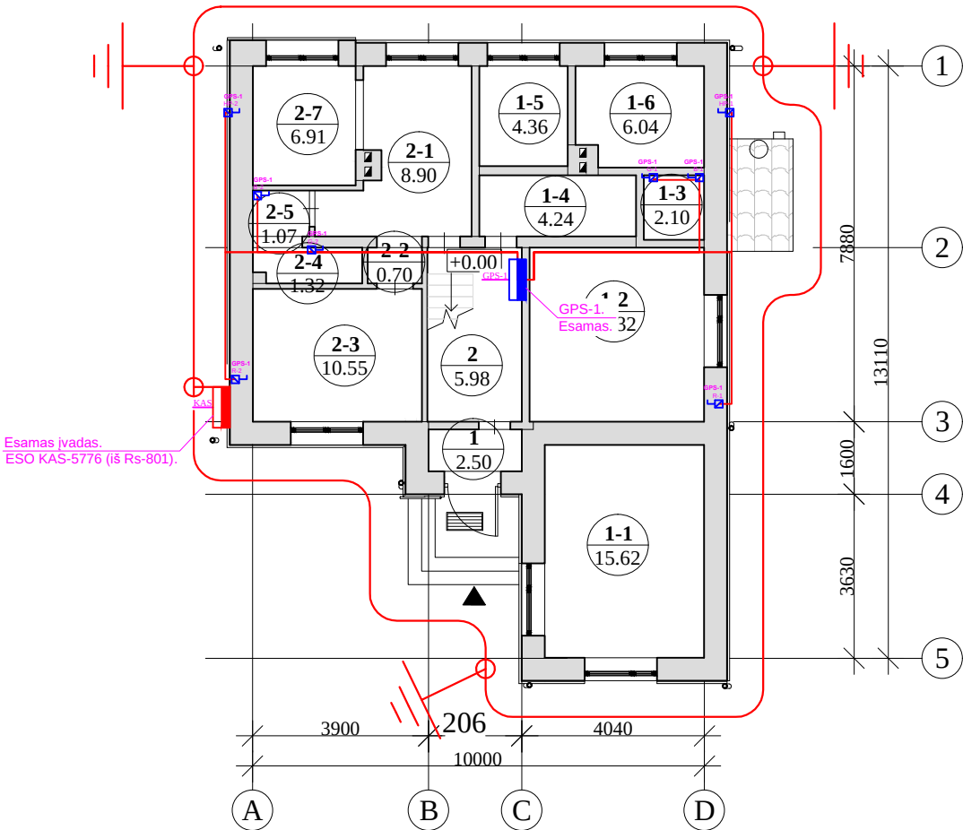
PIRMO AUKŠTO PLANAS
