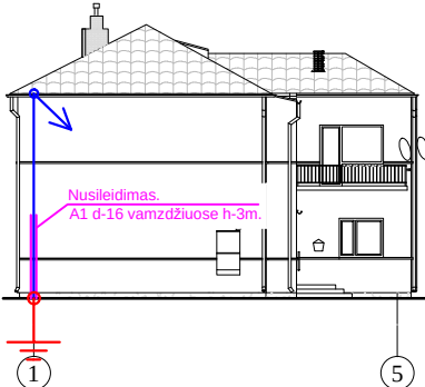
FASADAS TARP AŠIŲ 1-3
