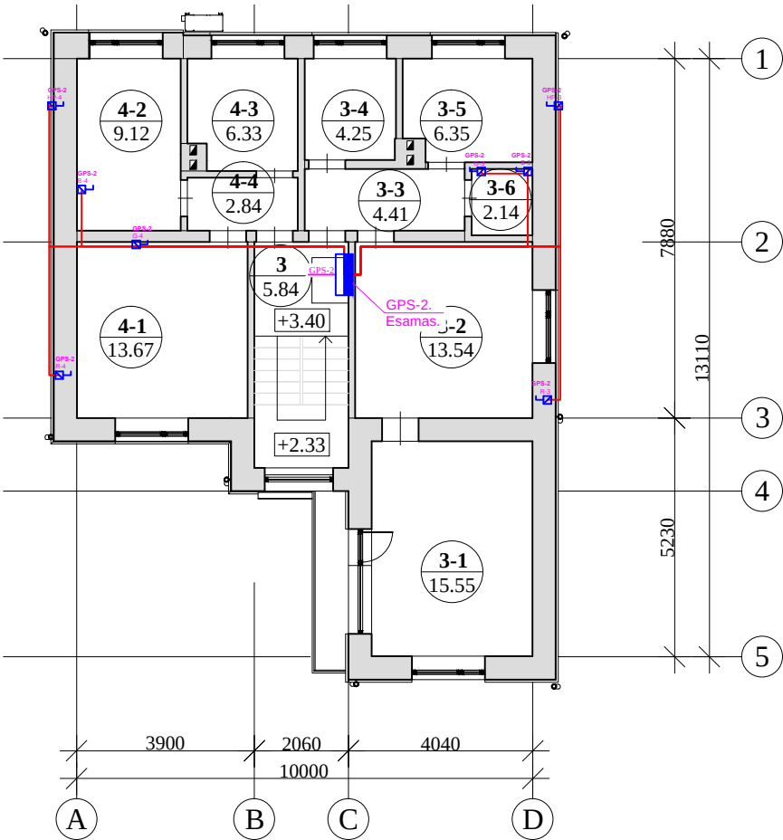
ANTRO AUKŠTO PLANAS
