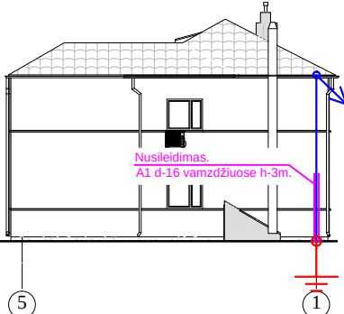
FASADAS TARP AŠIŲ 5-1
