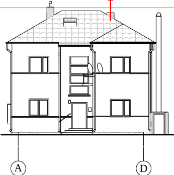
FASADAS TARP AŠIŲ A-D
